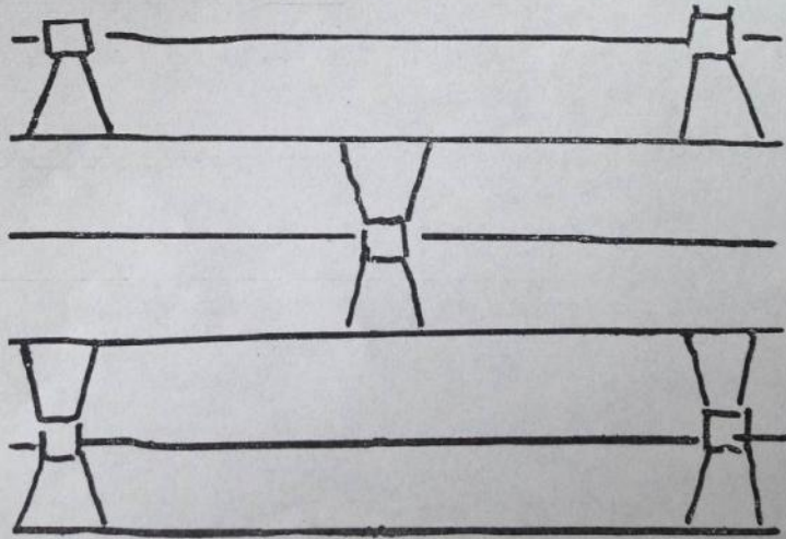
Levha IV/b — «Hâfânî Türk» mimârisinin alâmetlerinden biri olan ve Birinci İbrâhîm medresesinde de görülen, «kelebek»'ler ile ayrılmış, pişmiş tuğla dizmek tekniğinin schema'sı.
