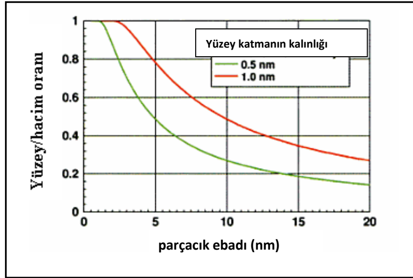
Şekil 2.6: Yüzey/hacim oranının parçacık ebadına göre değişimi [33,34]
