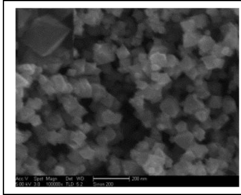
Şekil 2.14: Sentezlenmiş farklı büyüklükteki regular oktahedral Ni NP'nin SEM görüntüsü[40]
