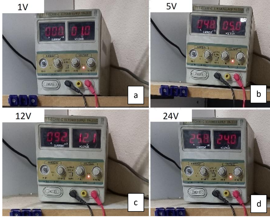
Şekil 5. 2. %11,7gr grafir Takviyeli biyoplastik elektriksel ölçümleri (a) 1Volt, (b) 5Volt, (c) 12Volt, (d) 24Volt.
