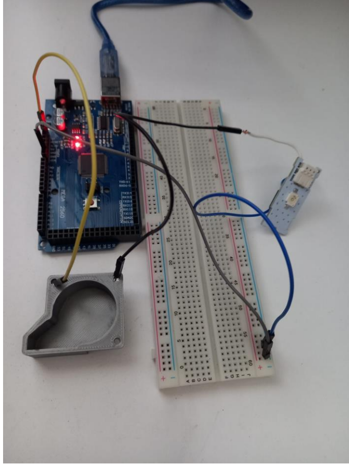
Şekil 5. 16. PLA biyoplastiğın elektriksel iletim deneyi.
